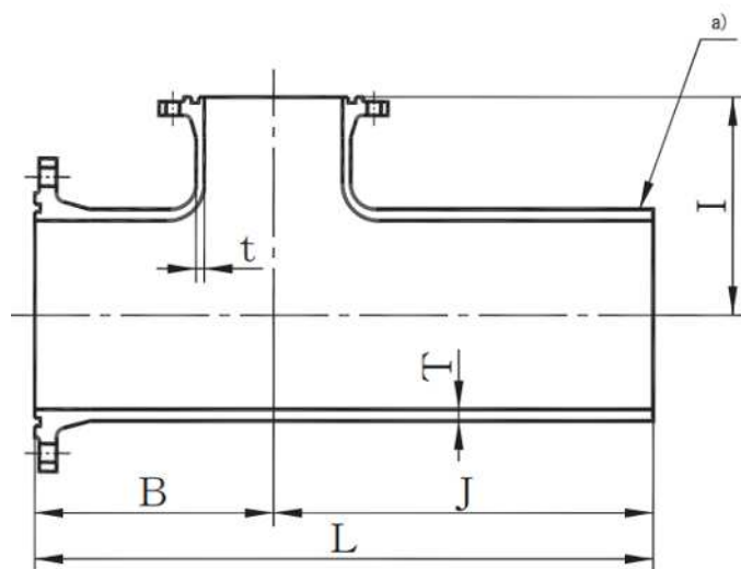
a)挿し口はK形による
